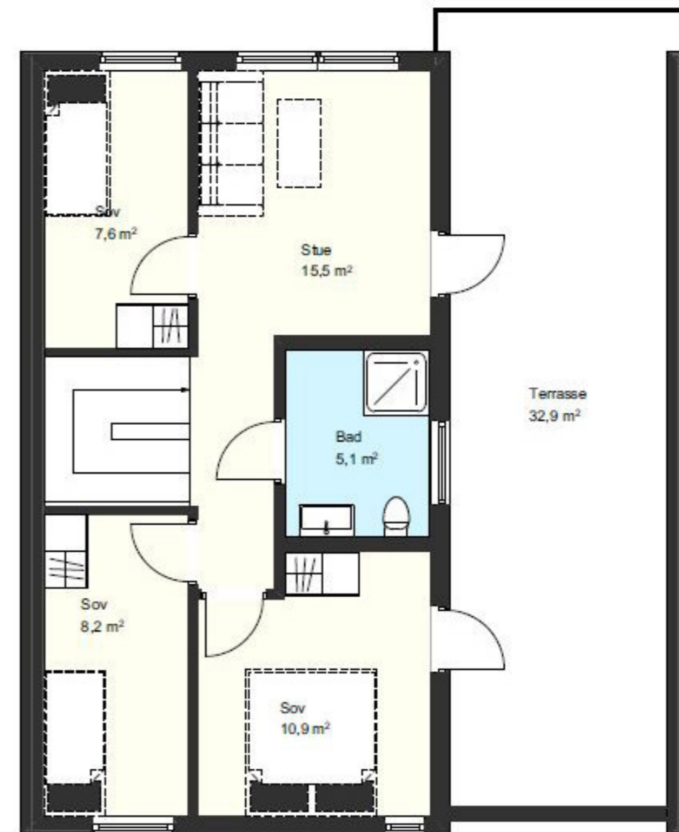
2. etasje i Kløverhagen hus C-F med seksjon 7-20
